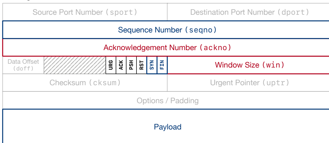
TCPSegment
